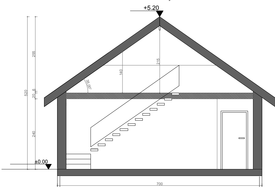
PRZEKRÓJ
