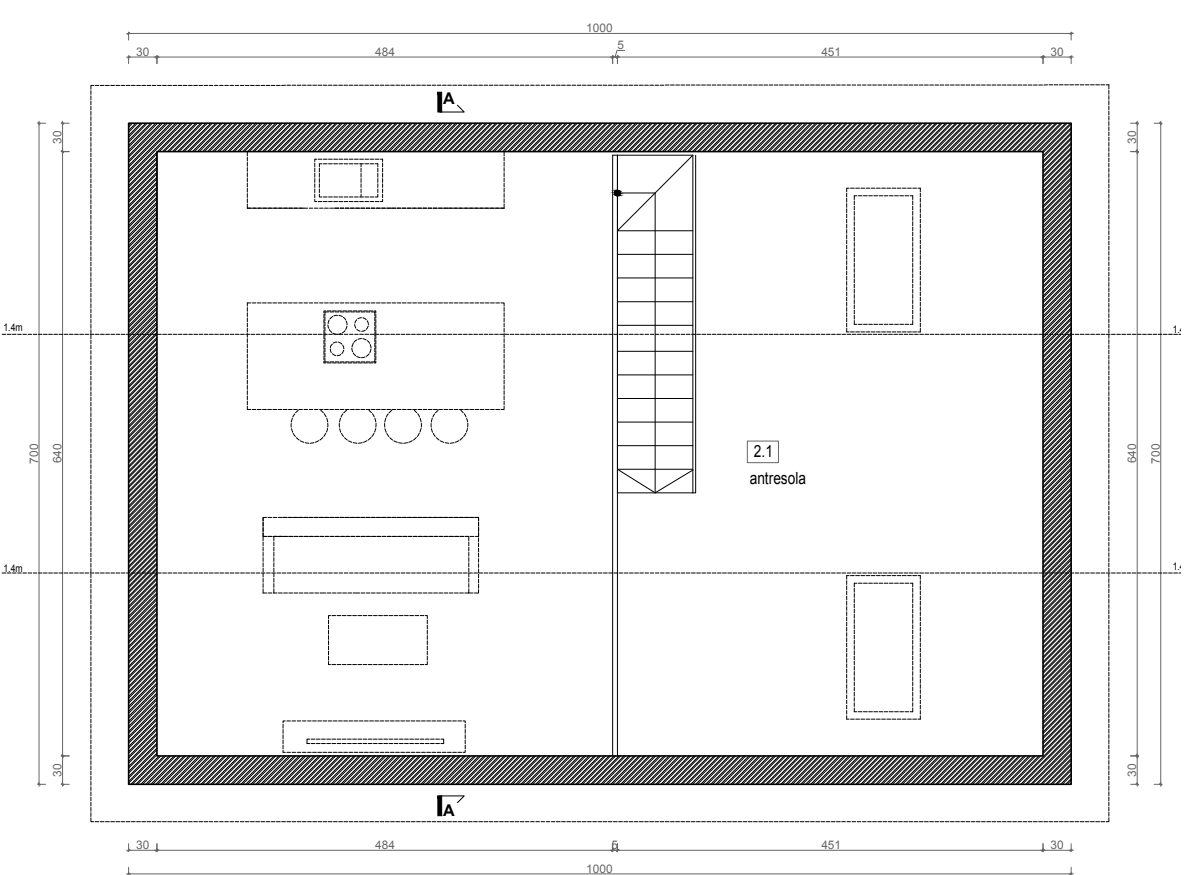
RZUT WARIANT Z ANTRESOLĄ
