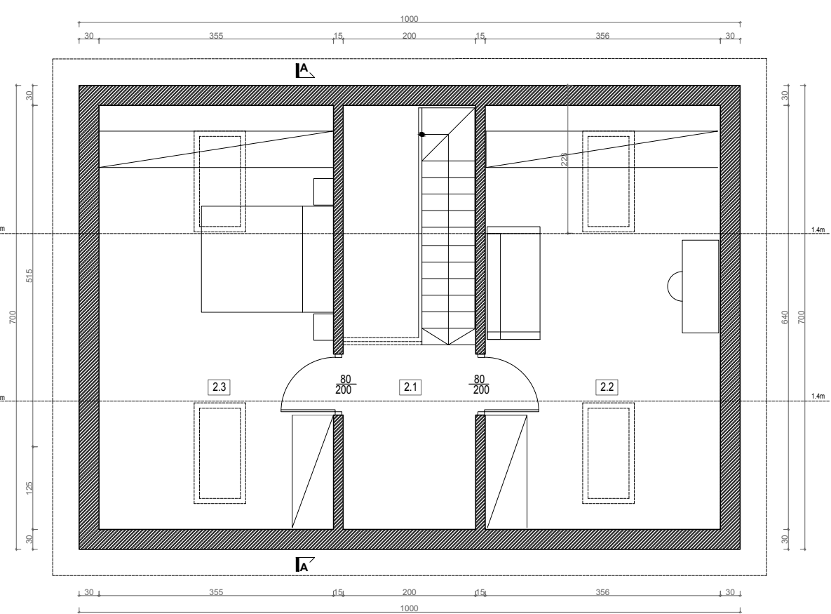
RZUT WARIANT Z Poddaszem
