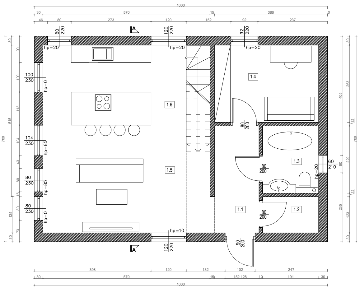
RZUT PARTERU
